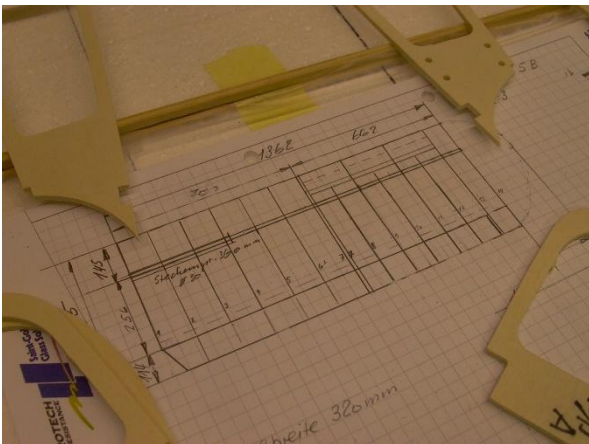
Selbsterstellter sehr einfacher Tragflächenplan und Bau in der Styrohelling.
